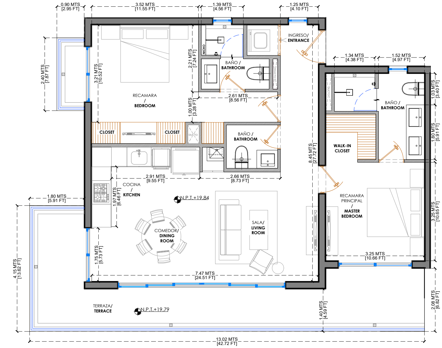
ESCALA 1:75
