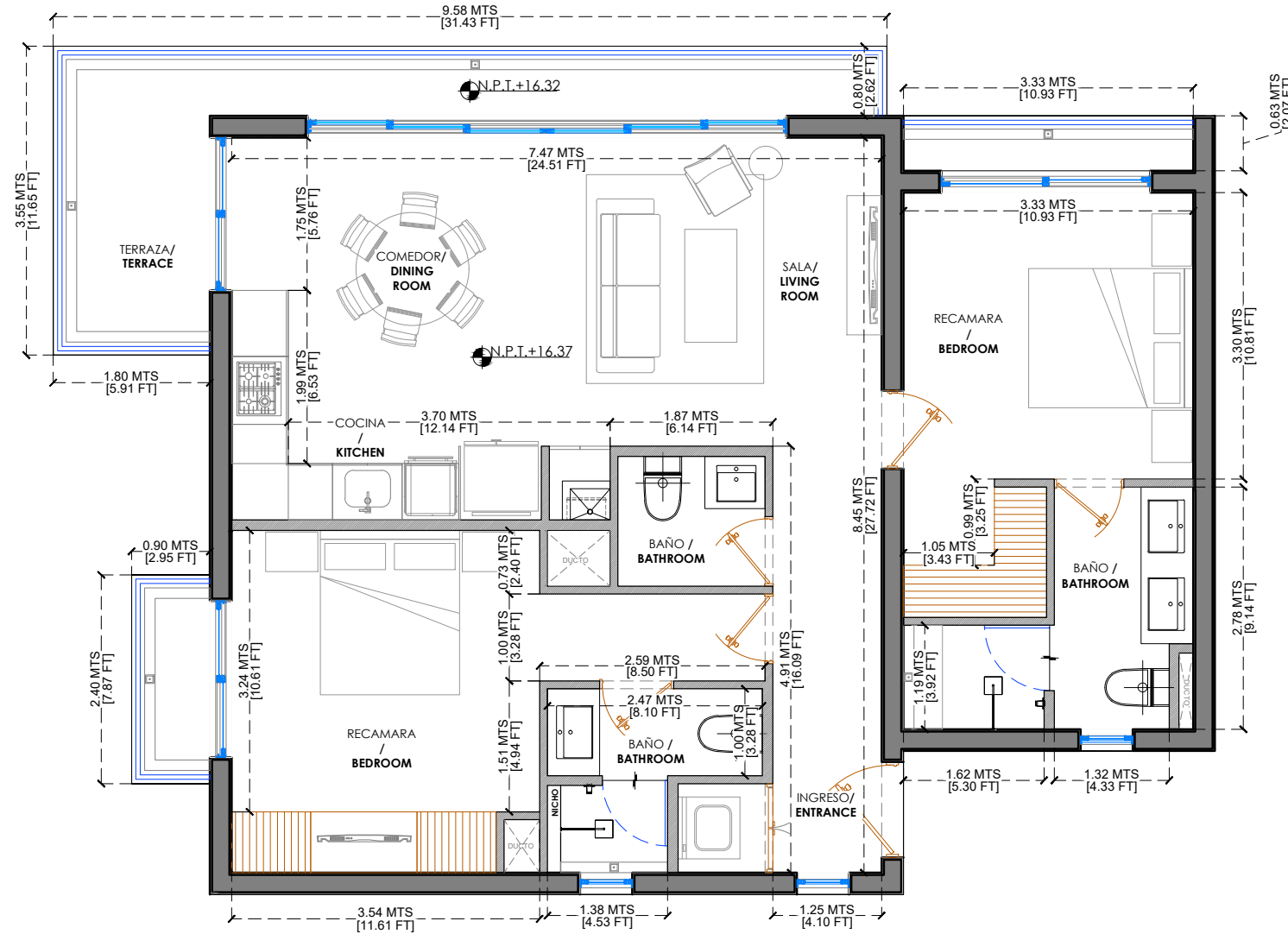
ESCALA 1:75
