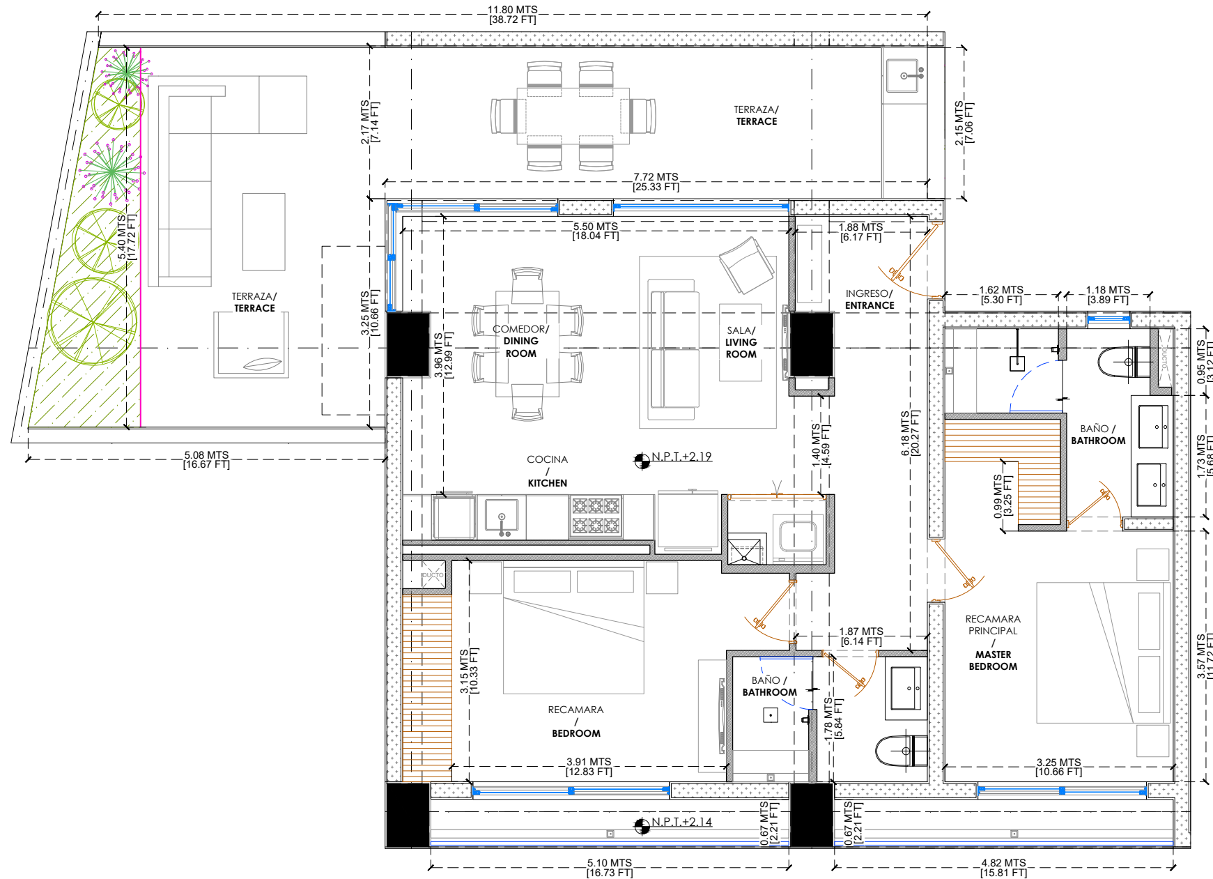
ESCALA 1:75
