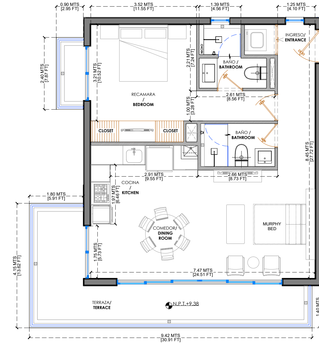
ESCALA 1:75
