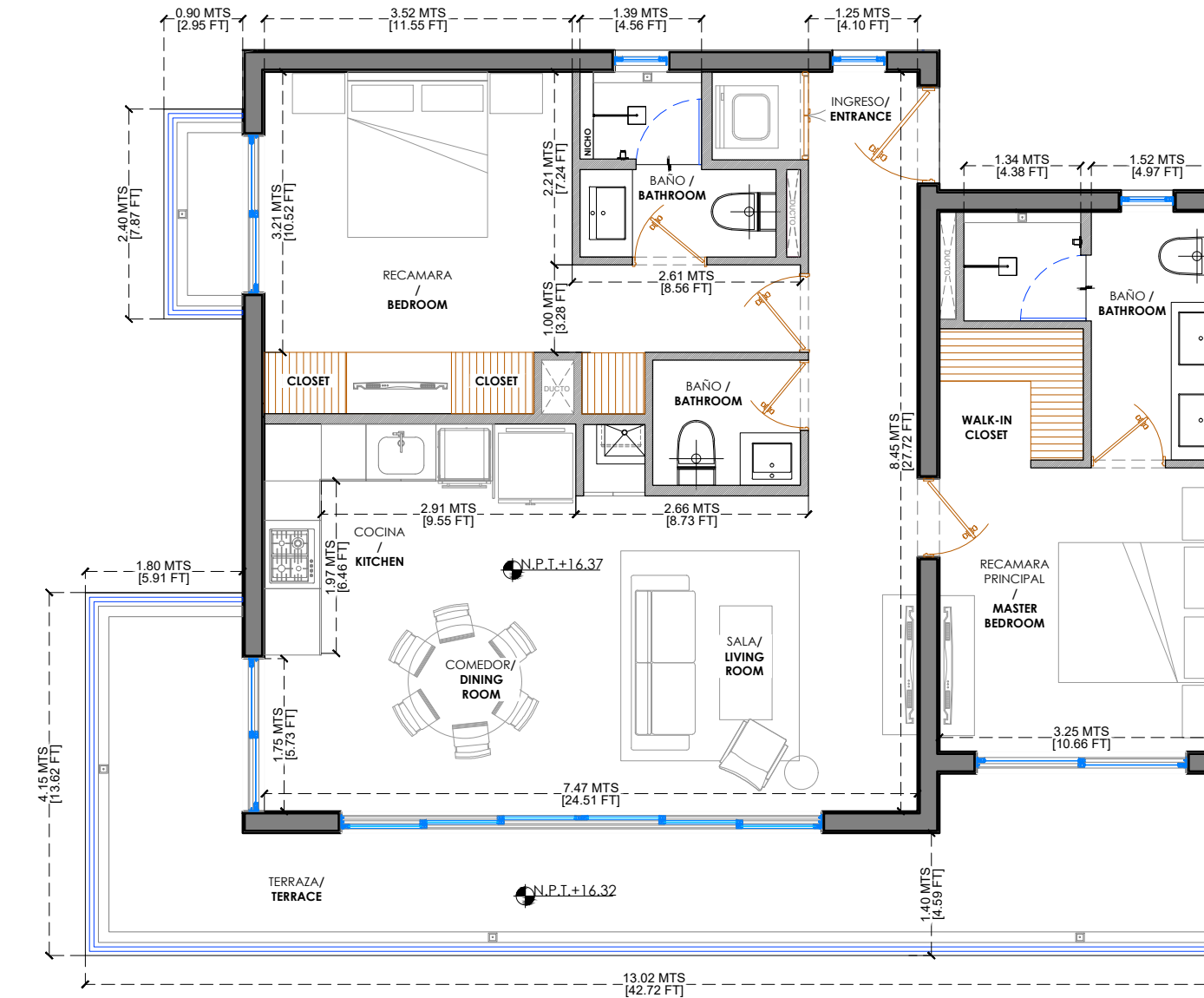
ESCALA 1:75
