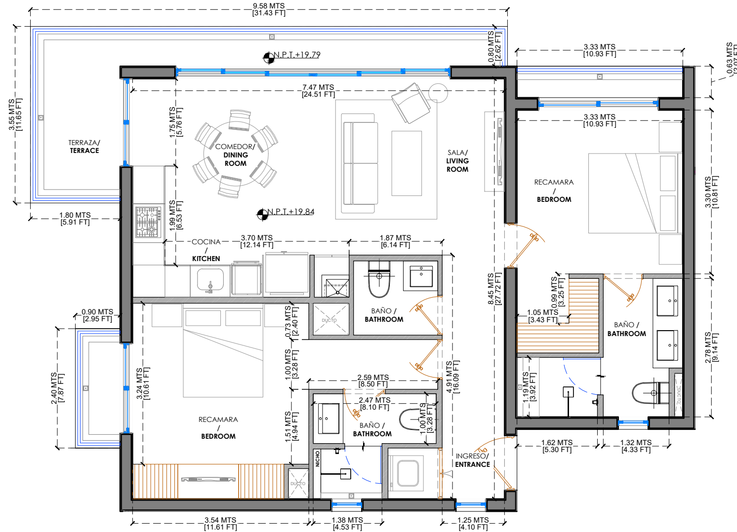
ESCALA 1:75
