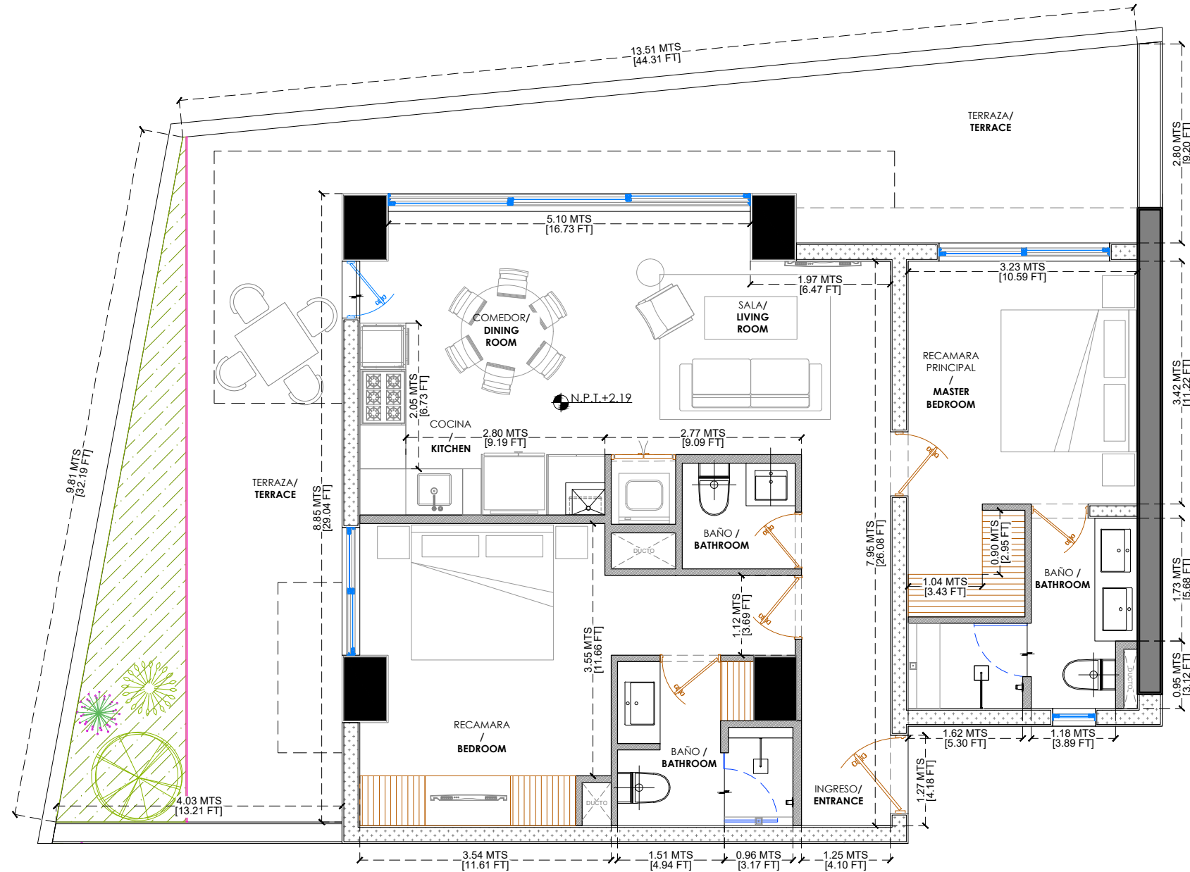
ESCALA 1:75
